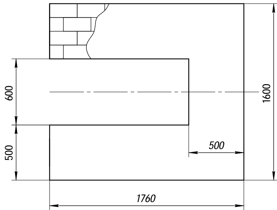
Основание котла (рекомендуемое)
